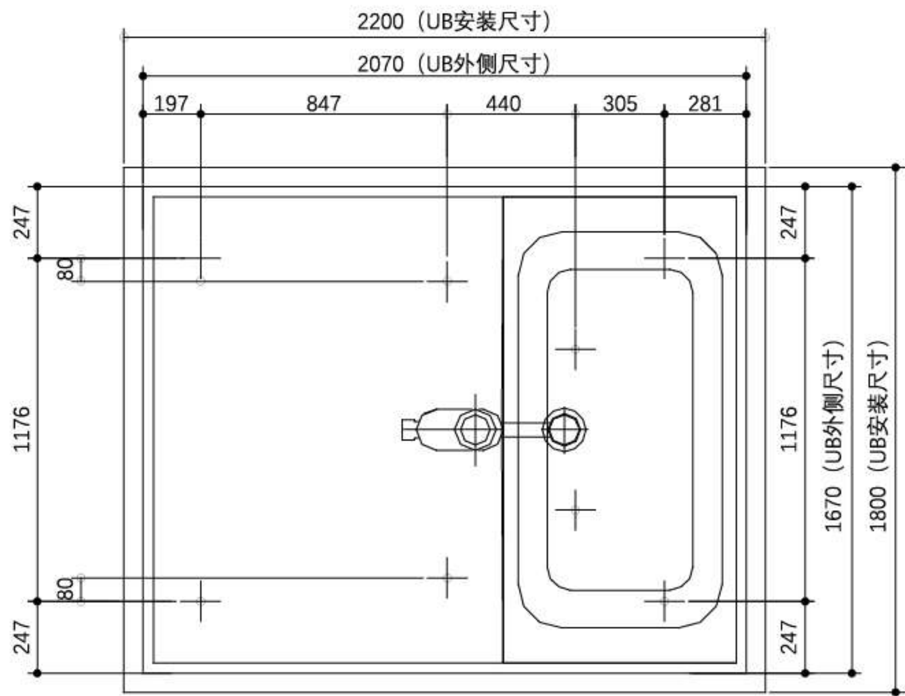
地脚安装位置图
