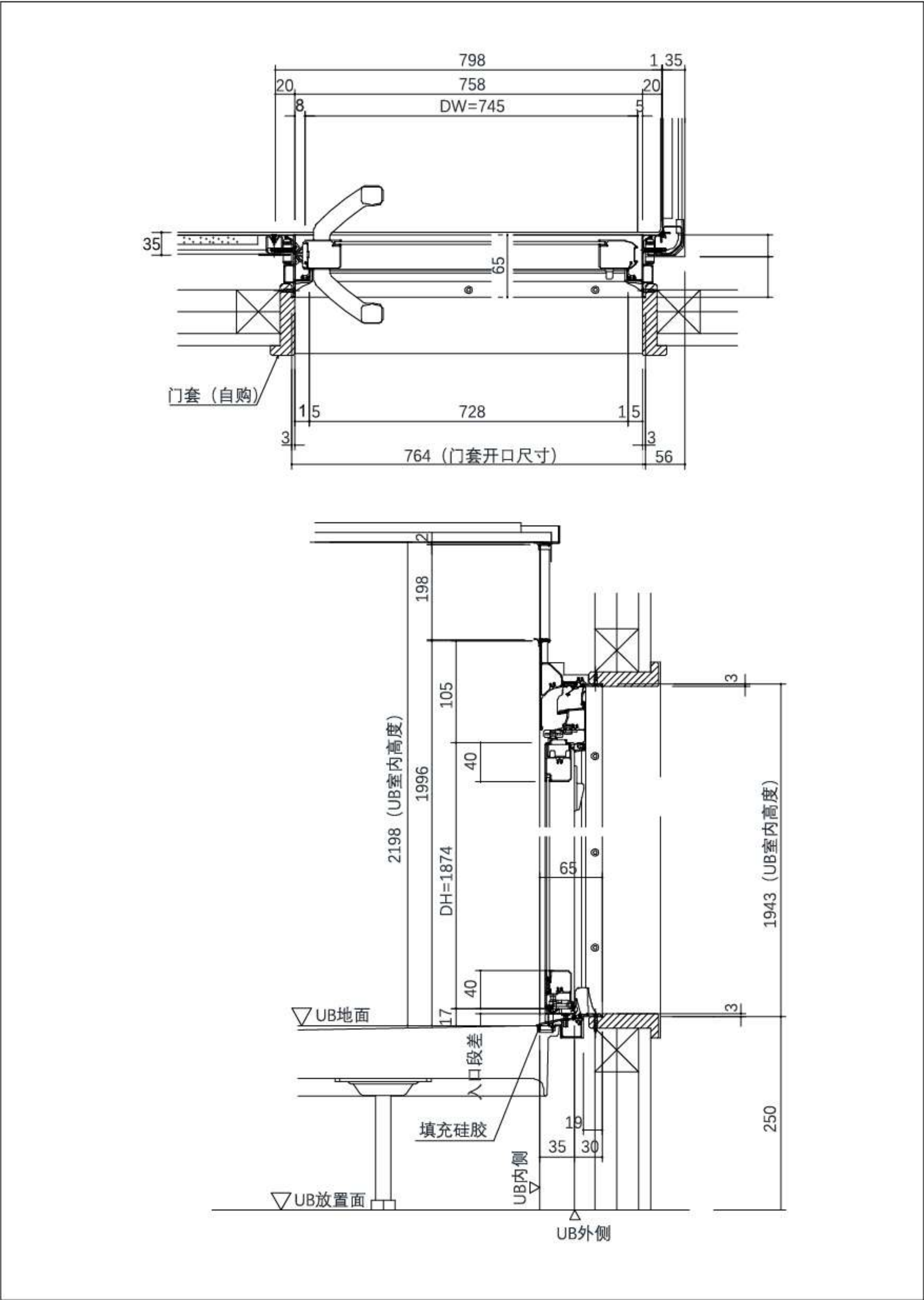
平开门详细图
