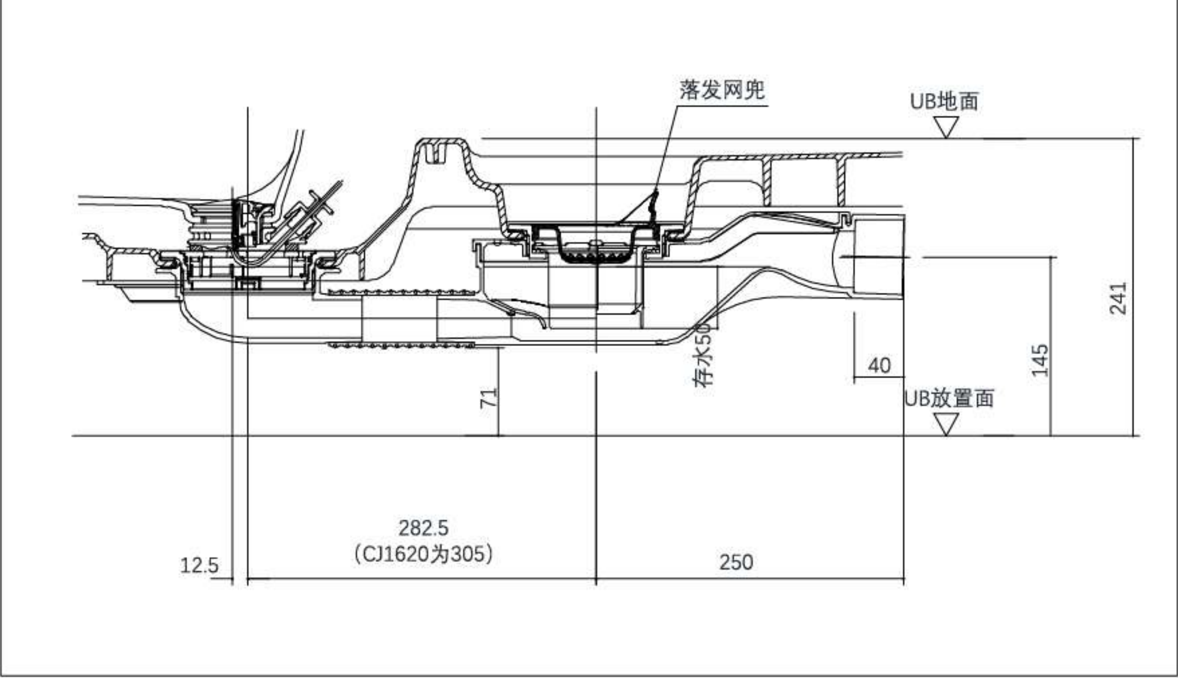
地漏详细图
