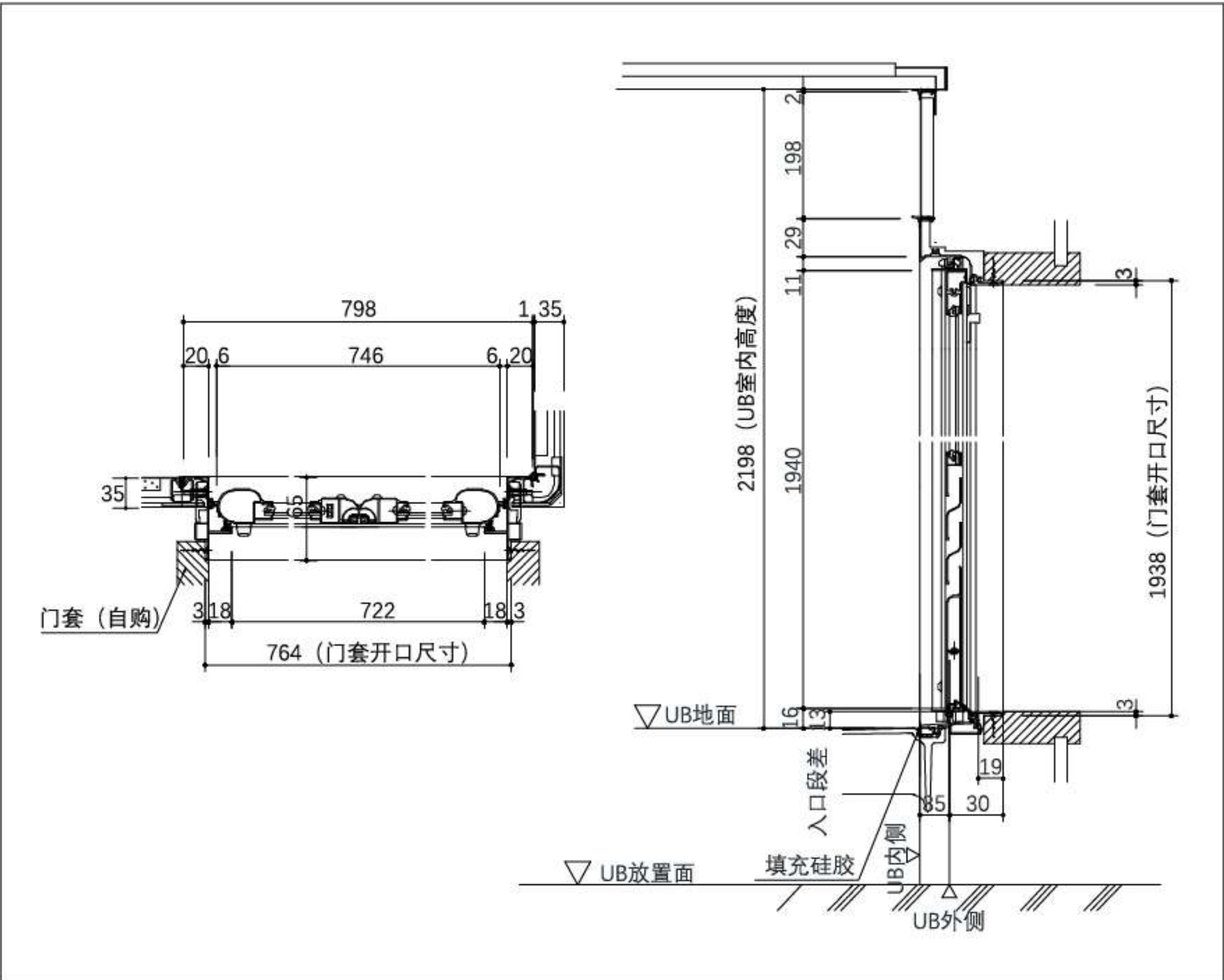
折叠门详细图
