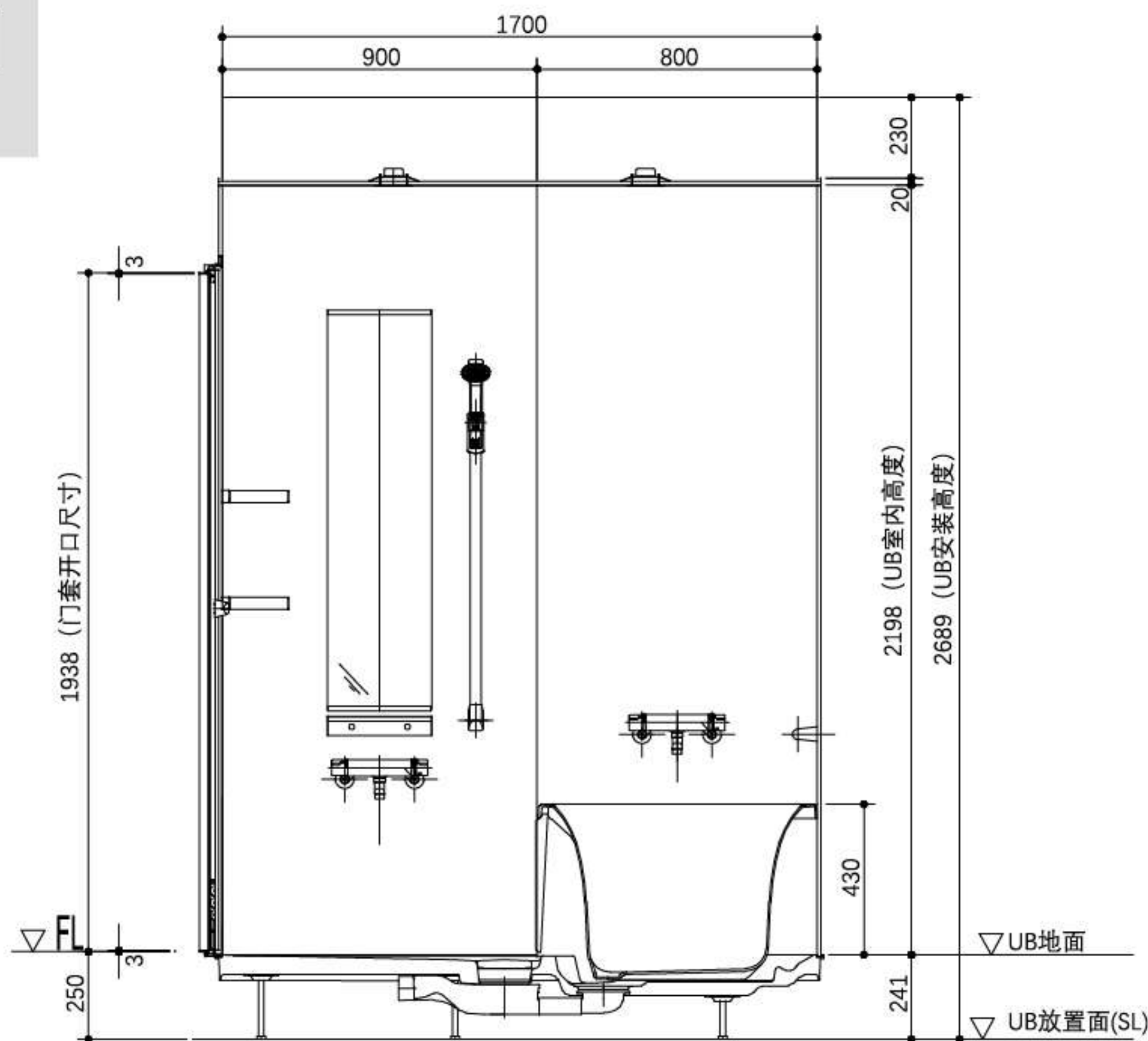
立面图 (长边)
