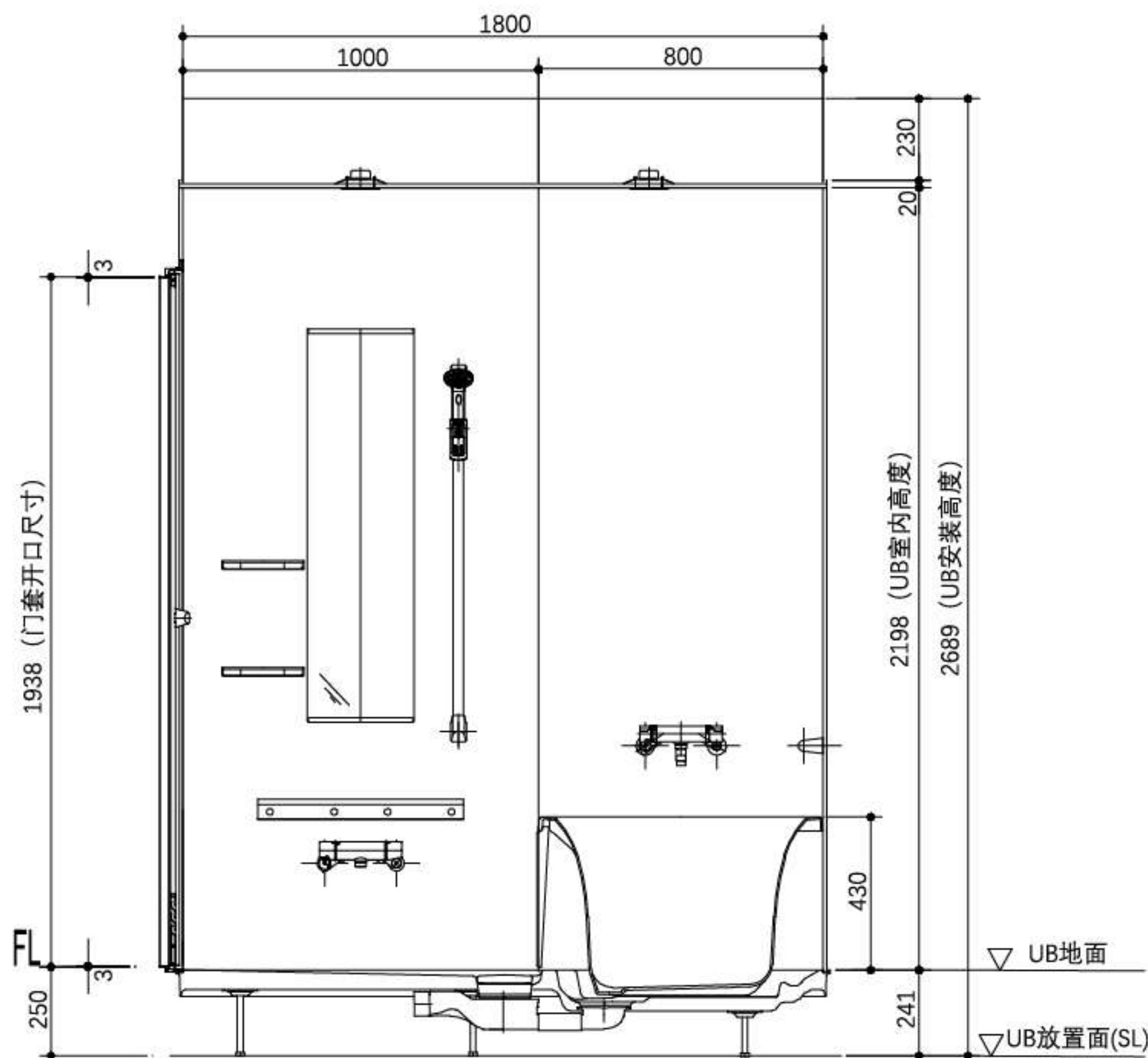
立面图 (长边)
