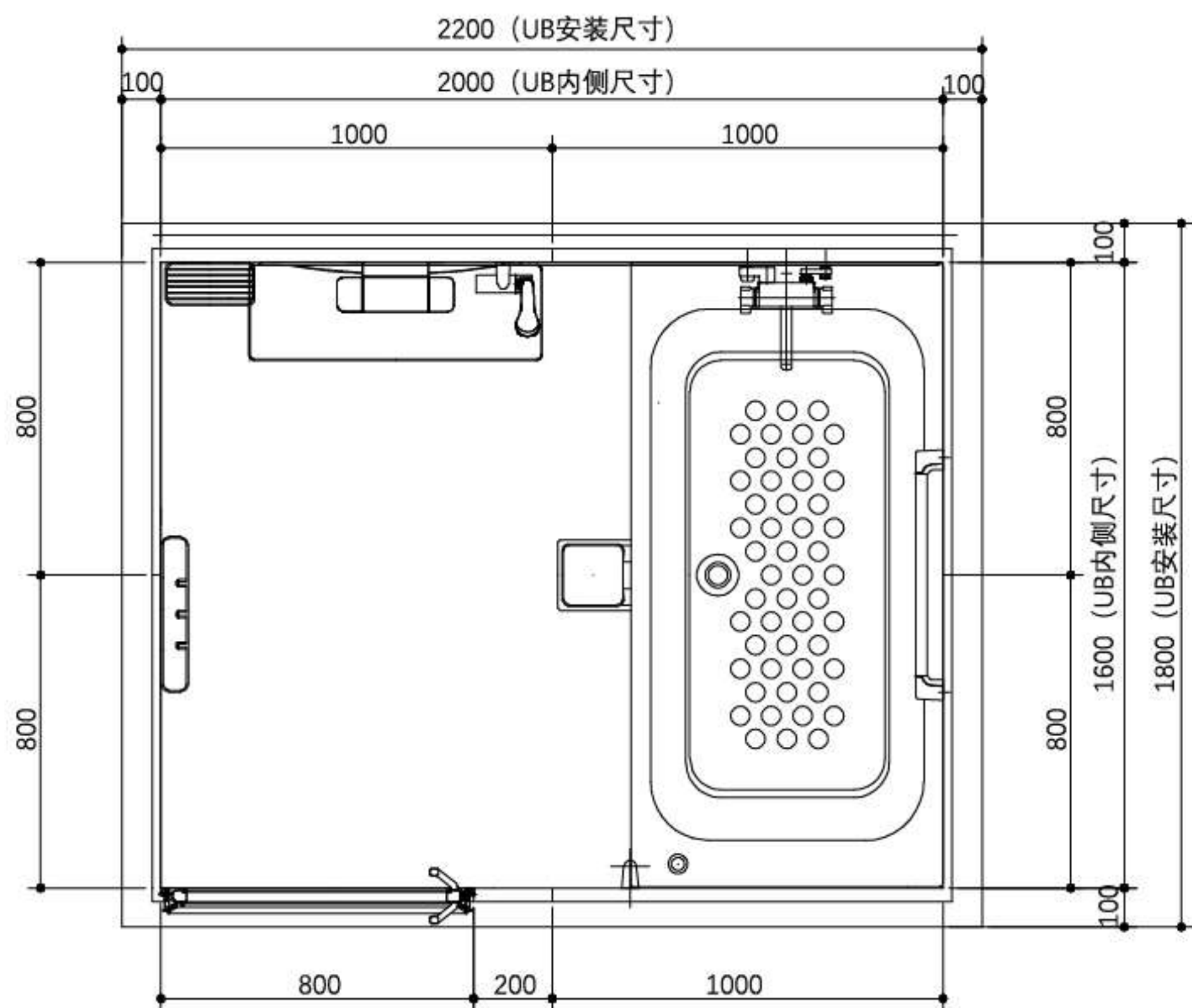
平面图
